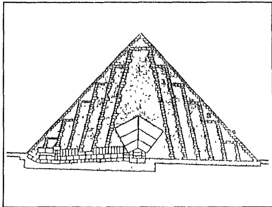
شكل (١٩) عقود التحفيف في هرم ساحو رع، باني صير ١ - كتل النواه ٢ - السطوح الداخليه ٣ - الكتل الرابطة ٤ - كتل الكسوة من
